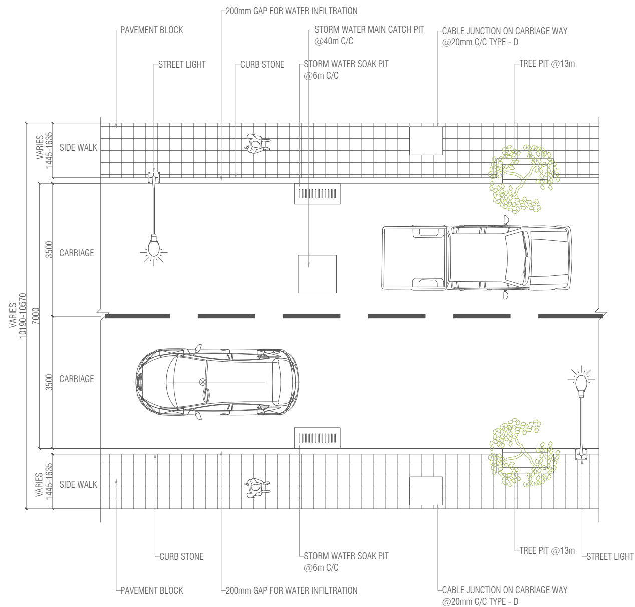
KALEYFAANU MAGU - PLAN 1:100
