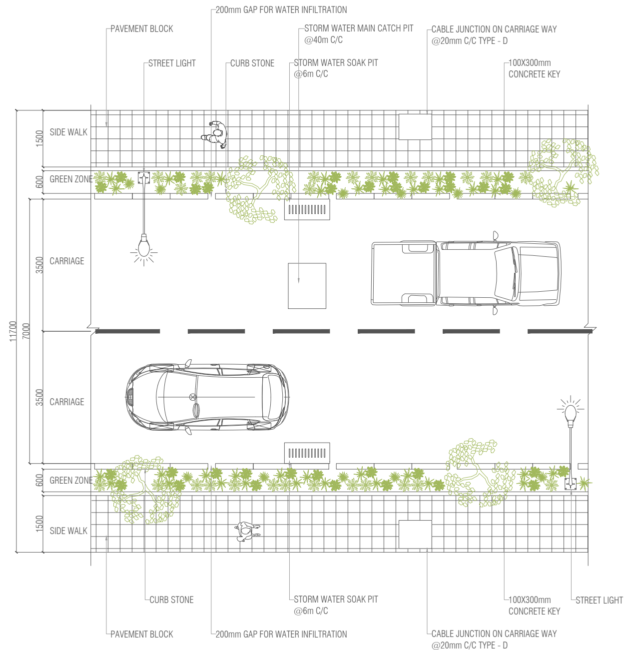
INJEENUGEY DHEKONU MAGU - PLAN 1:100
